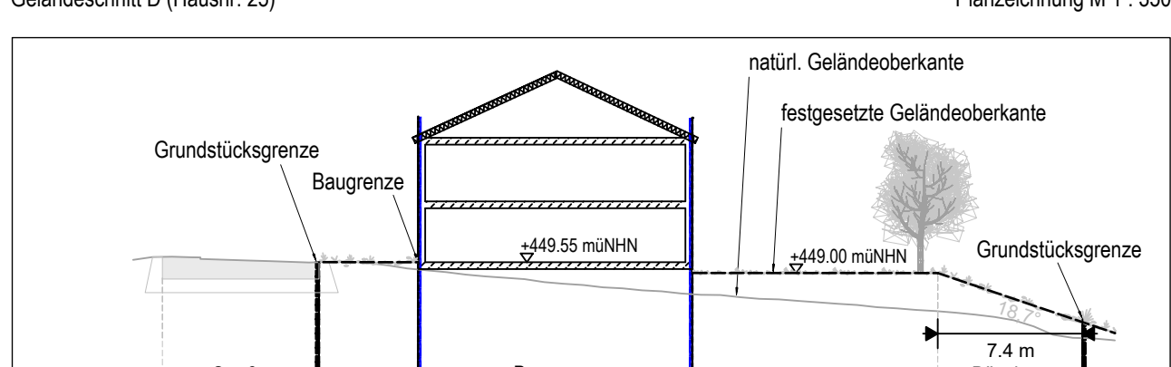
Geländeschnitt E (Hausnr. 27) Planzeichnung M 1 : 350
