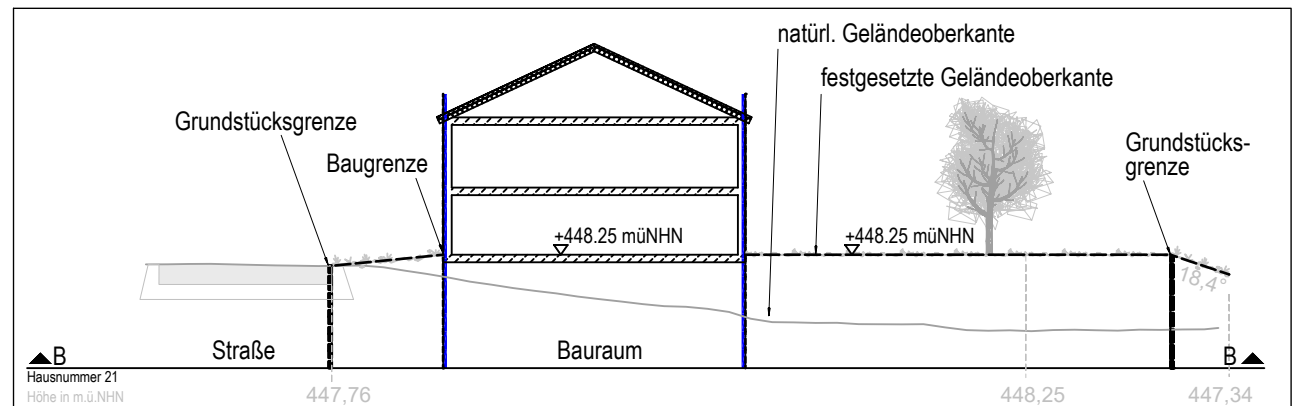
Geländeschnitt B (Hausnr. 21) Planzeichnung M 1 : 350
