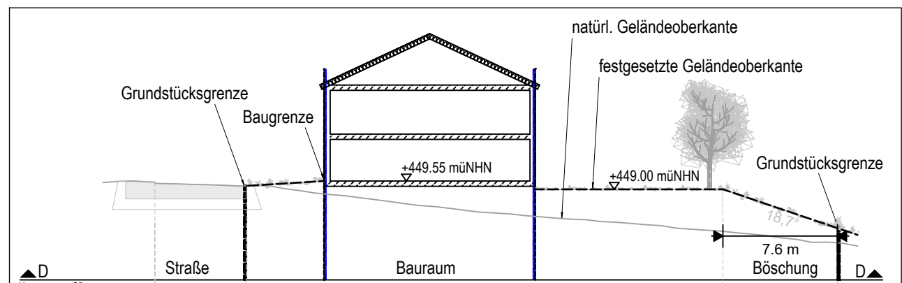
Geländeschnitt D (Hausnr. 25) Planzeichnung M 1 : 350
