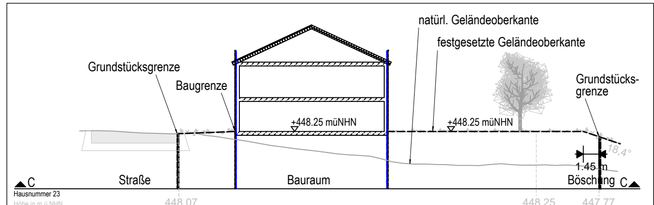
Geländeschnitt C (Hausnr. 23) Planzeichnung M 1 : 350
