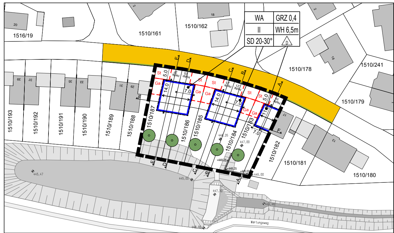
Geobasisdaten: Bayerische Vermessungsverwaltung Planzeichnung M 1 : 1000
