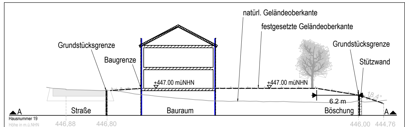
Geländeschnitt A (Hausnr. 19) Planzeichnung M 1 : 350
