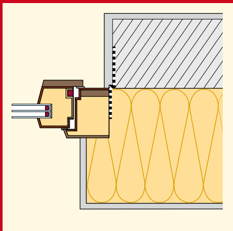
Querschnitt: Massivbauweise | Holzbauweise
