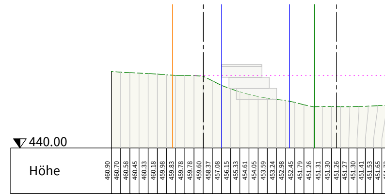
Geländeschnitt 8 - 8
