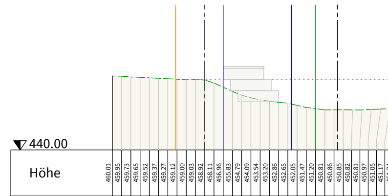
Geländeschnitt 9 - 9
