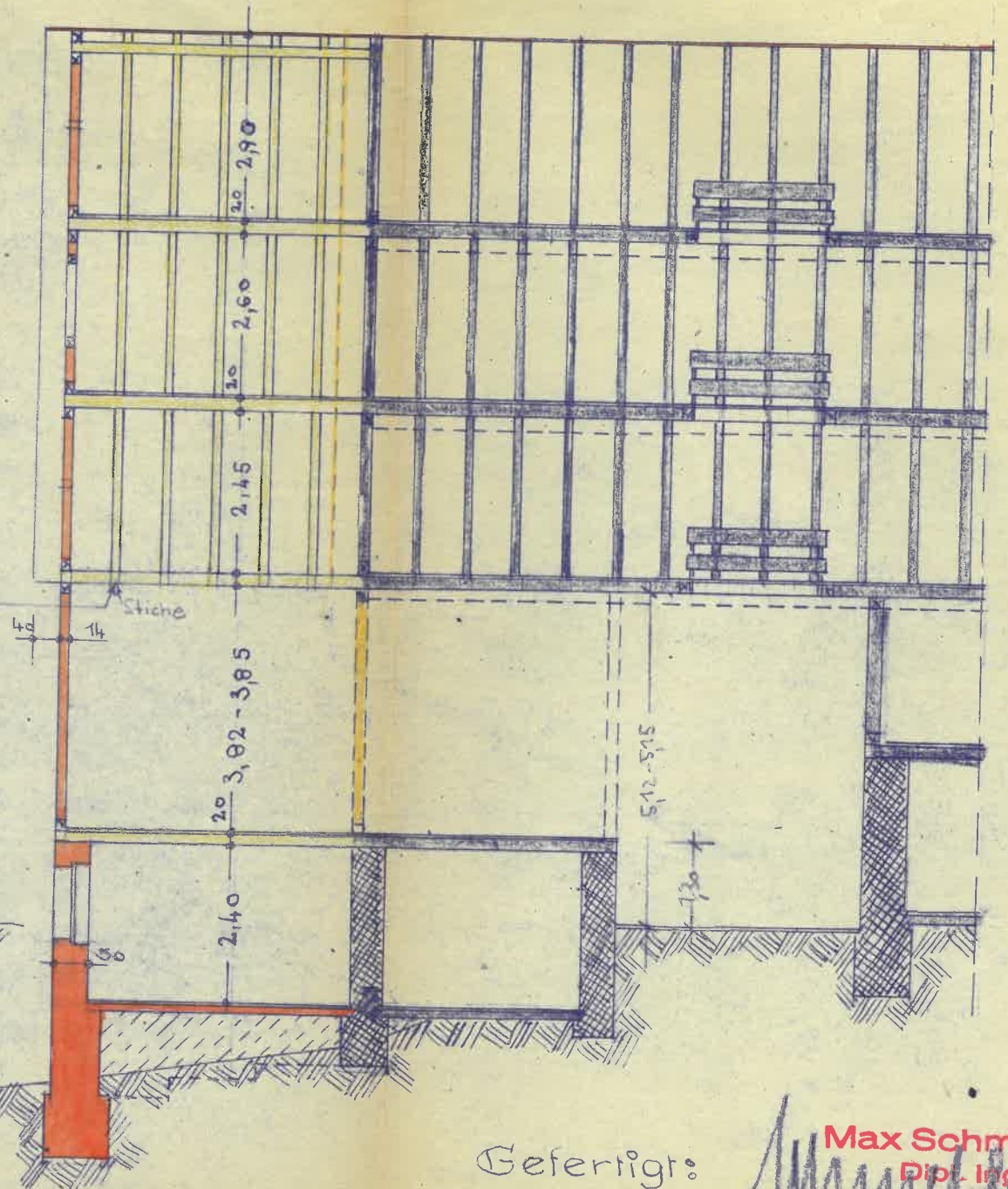
Längenschnitt.
