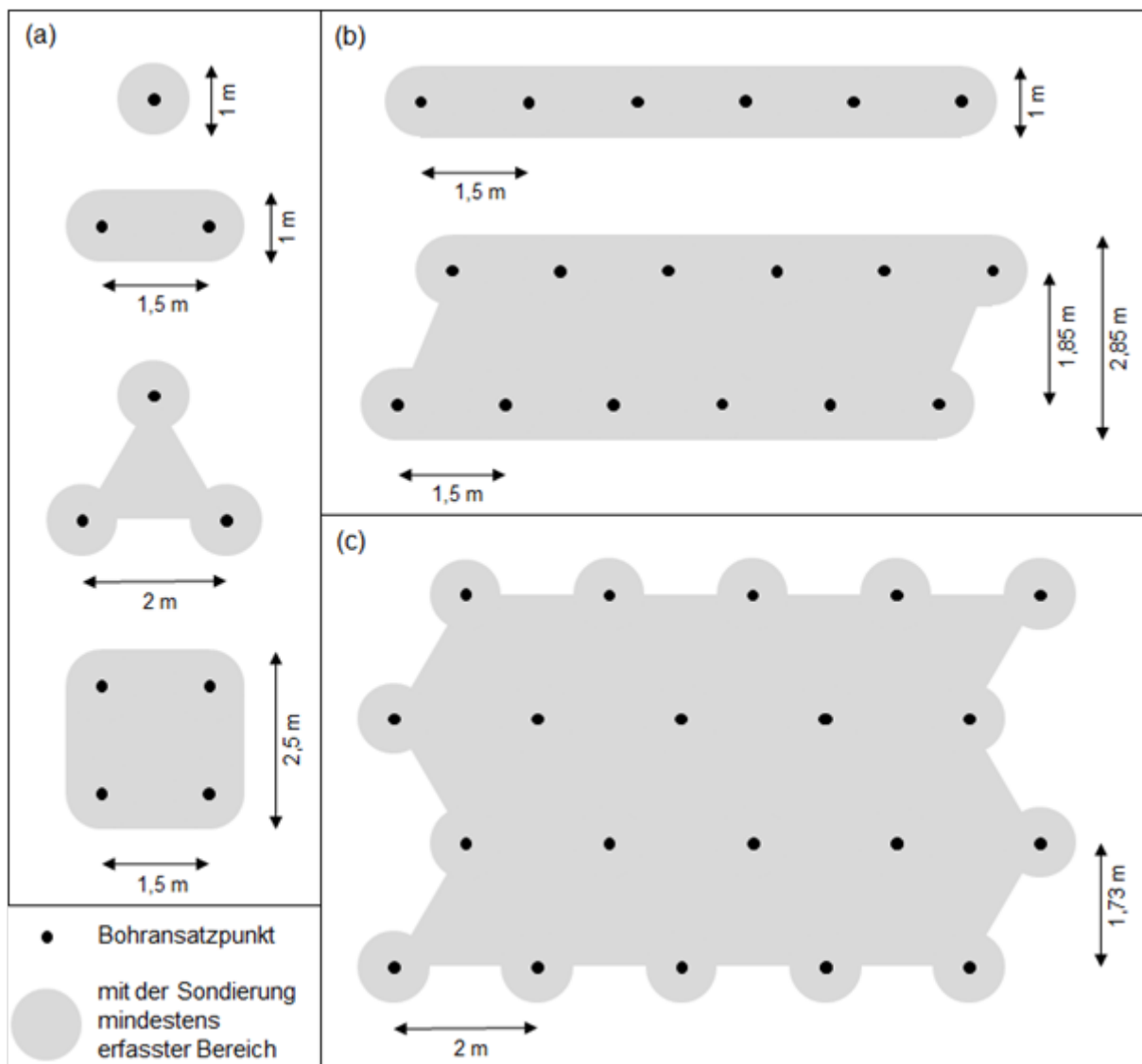
Abbildung 1 – Standard-Bohrlochraster für (a) punkartige (b) linienförmige und (c) flächige Untergrunderkundungen (ersetzt keine Flächenüberprüfung) mittels geomagnetischer Bohrlochdetektion.
