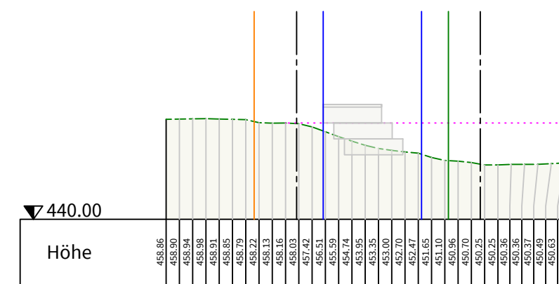
Geländeschnitt 10 - 10
