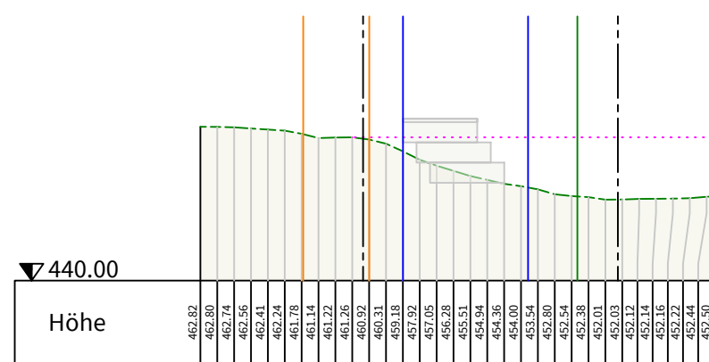
Geländeschnitt 6 - 6
