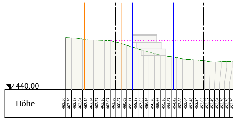
Geländeschnitt 5 - 5
