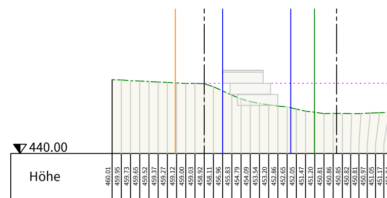
Geländeschnitt 9 - 9
