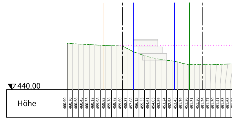
Geländeschnitt 8 - 8
