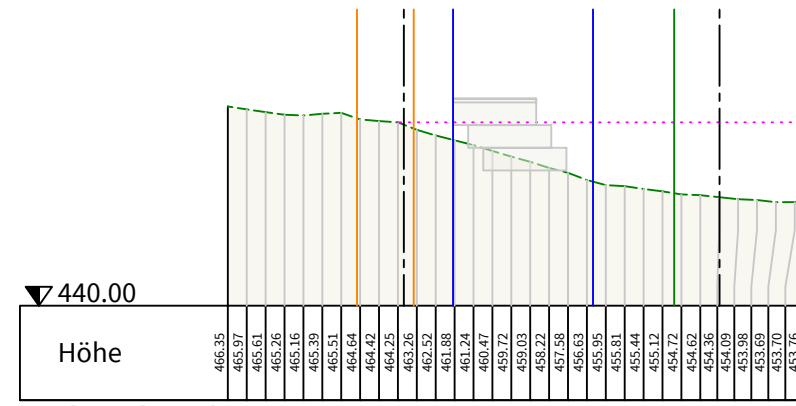
Geländeschnitt 2 - 2
