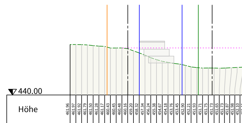
Geländeschnitt 7 - 7
