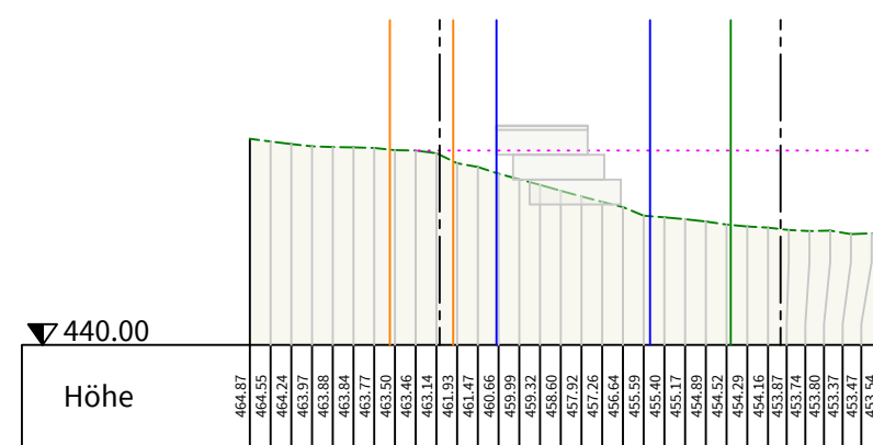
Geländeschnitt 3 - 3
