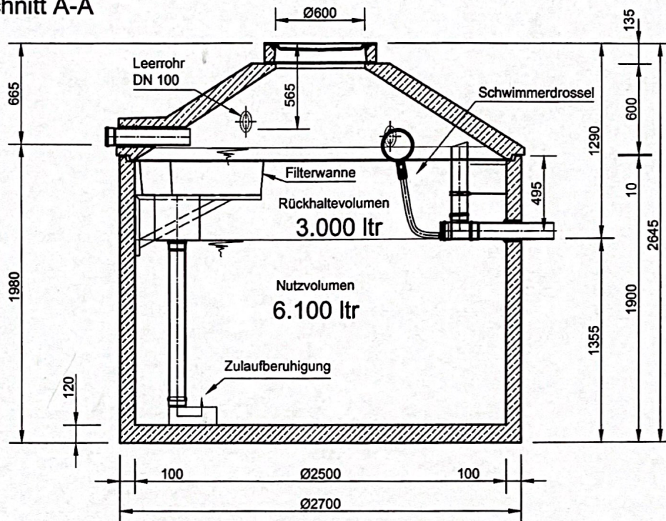
Schnitt A-A
