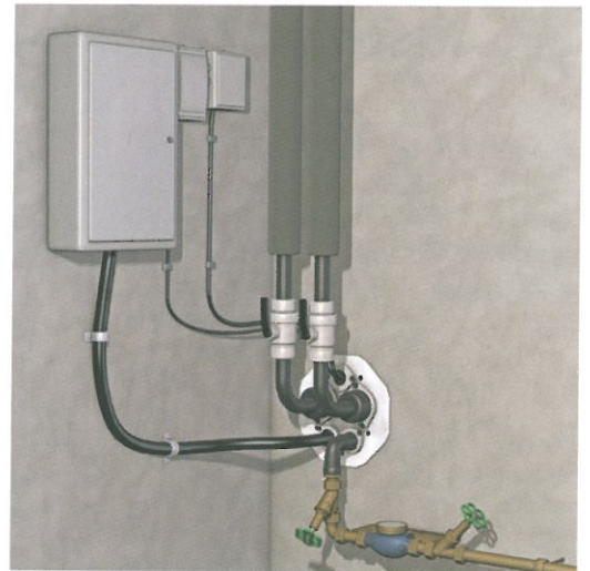
Mehrspartenhausanschluss mit Fernwärme
