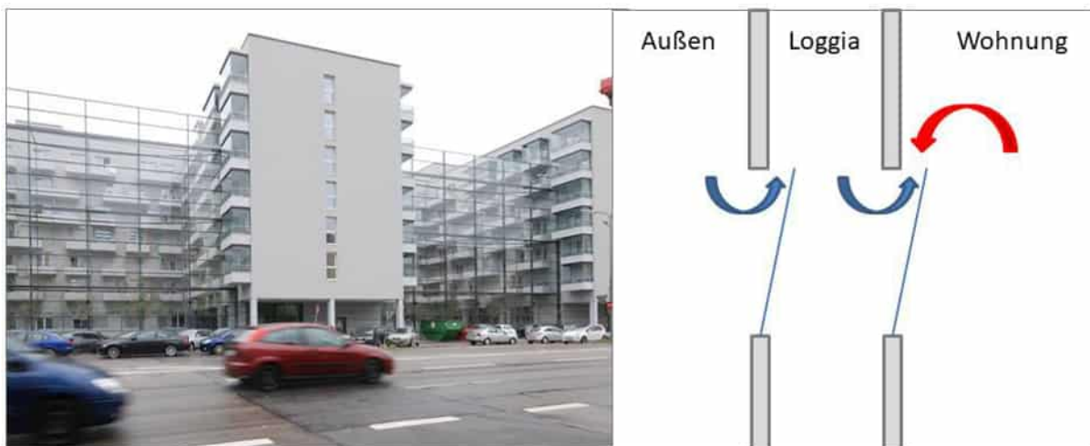
Abbildung 19: Verglaste Loggias in der Landsbergerstr. in München sowie schematische Darstellung der Belüftung
