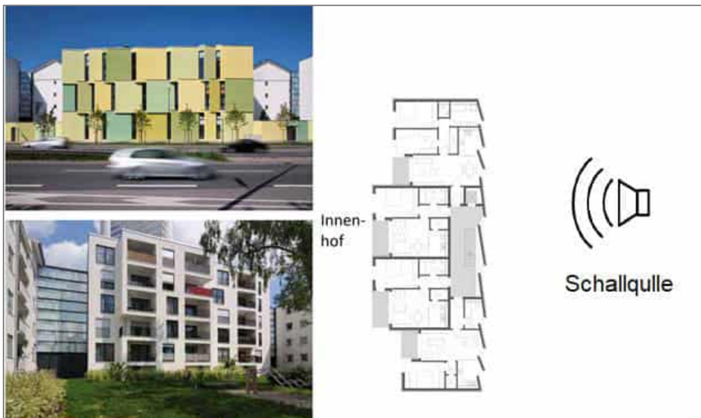
Abbildung 17: Beispiel geeigneter Grundrissgestaltung (Quelle: Endliche Ruhe, Neues Wohnen am Mittleren Ring, Landeshauptstadt München, August 2012);
