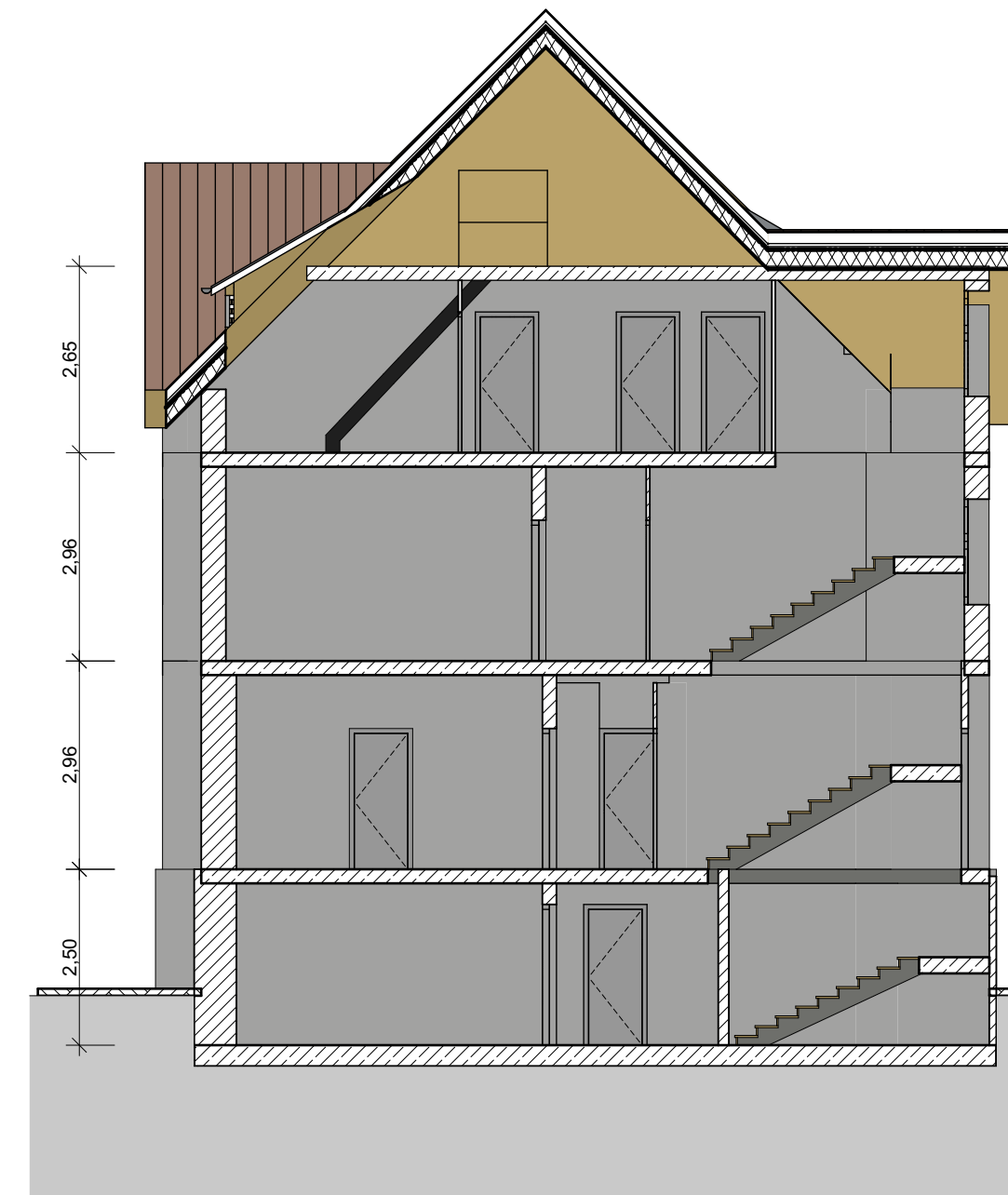
Schnitt
