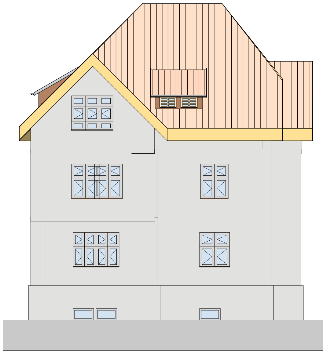
Südansicht
