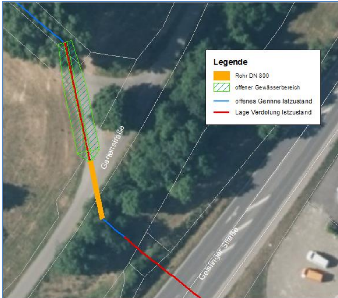
Abbildung 9: Erstellung Planzustand 2 – Lage des geöffneten Gerinneabschnitts des Klingelgrabens und der Verdolung Gartenstraße mit DN 800
